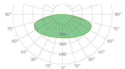
Diagramm: Lichtstreuung
